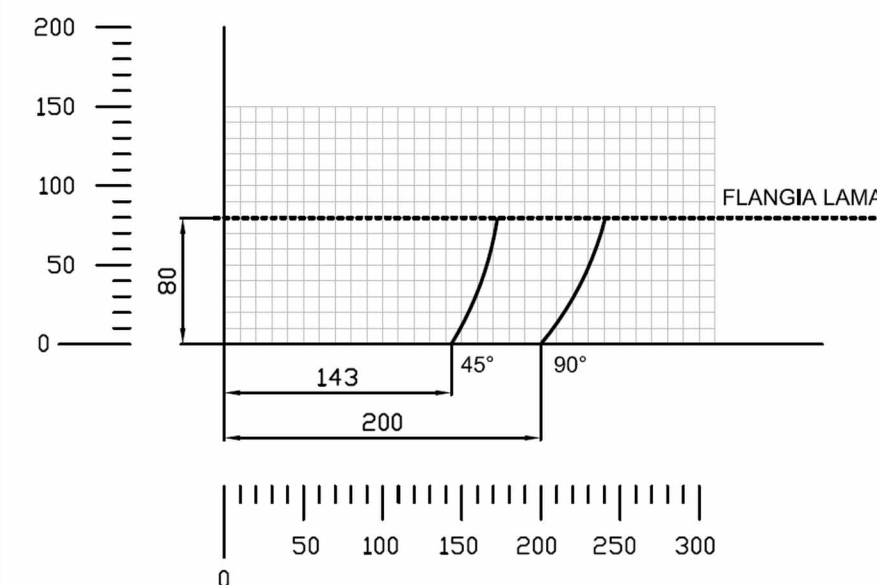
DIAGRAMMA DI TAGLIO TRONCATRICE MONO TESTA PENDOLARE VENUS400 (tolleranza \pm 3\text{mm} )
