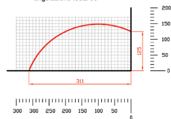
DIAGRAMMA DI TAGLIO TRONCATRICE ASCENDENTE LUNA CON LAMA Ø450mm E SQUADRO ARRETRATO DI 100mm
