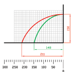
DIAGRAMMA DI TAGLIO TRONCATRICE ASCENDENTE LUNA CON LAMA Ø450mm
