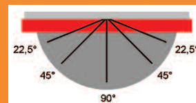
DIAGRAMMA DI TAGLIO TRONCATRICE ASCENDENTE LUNA CON LAMA Ø450mm
